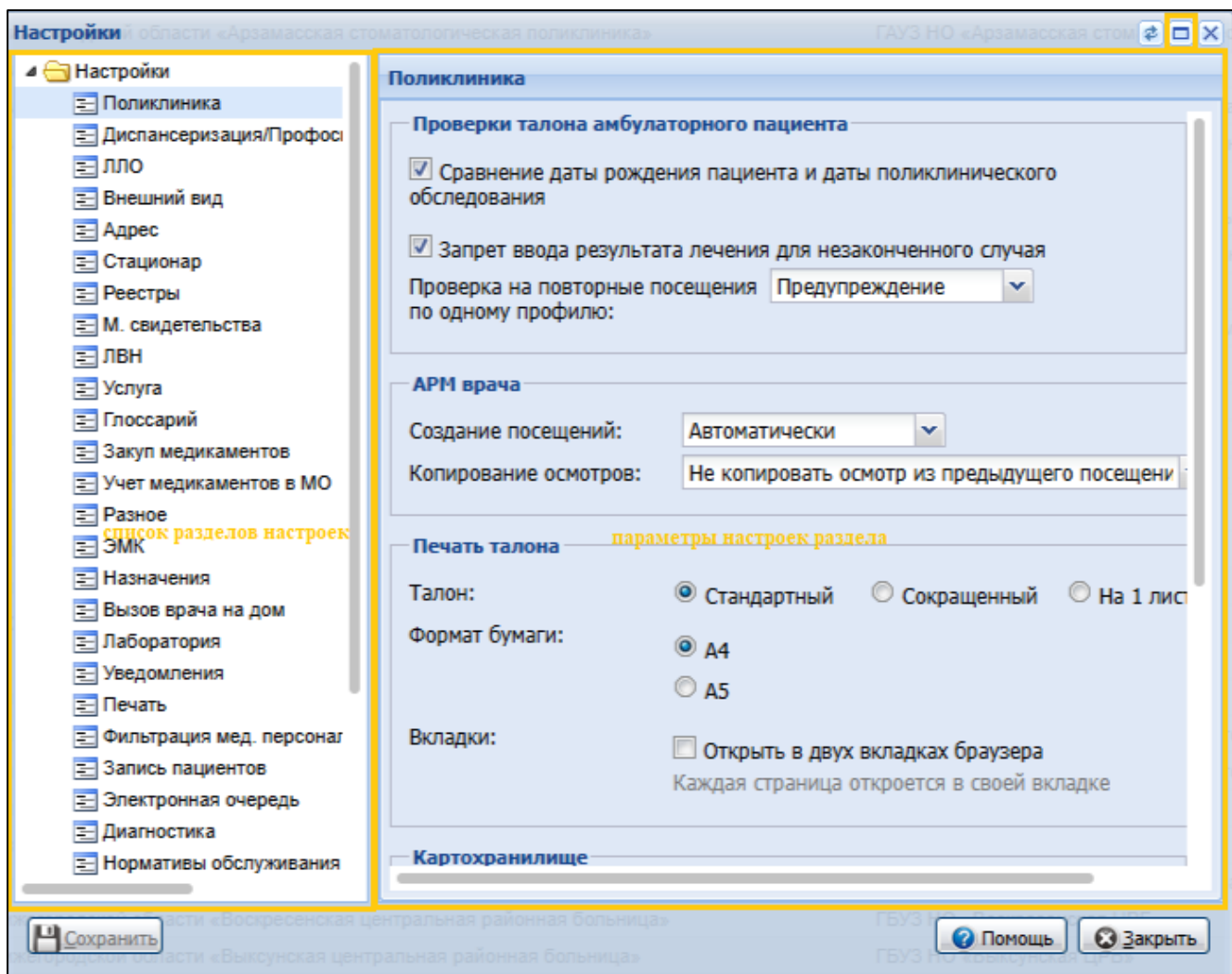
Рисунок 9 – Форма "Настройки"
