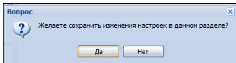
Рисунок 10 – Пример сообщения
